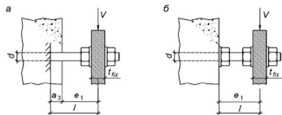
Рисунок 6.2 - Схема для определения плеча сдвигающей силы
