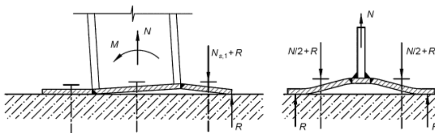
Рисунок 6.6 - Схема возникновения дополнительных усилий для гибких опорных плит
