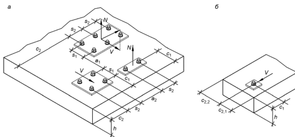
а - анкерная группа; б - одиночный анкер
