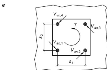
Рисунок 6.9 - Пример распределения сдвигающих усилий в анкерной группе при действии крутящего момента
