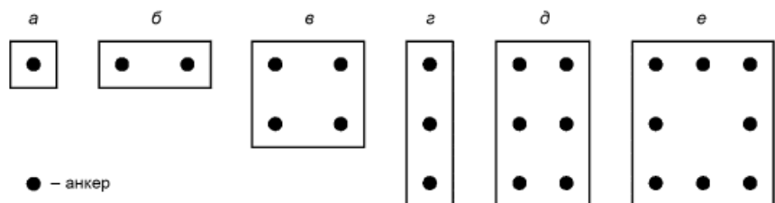
Рисунок 5.2 - Основные формы расстановки анкеров в группе
