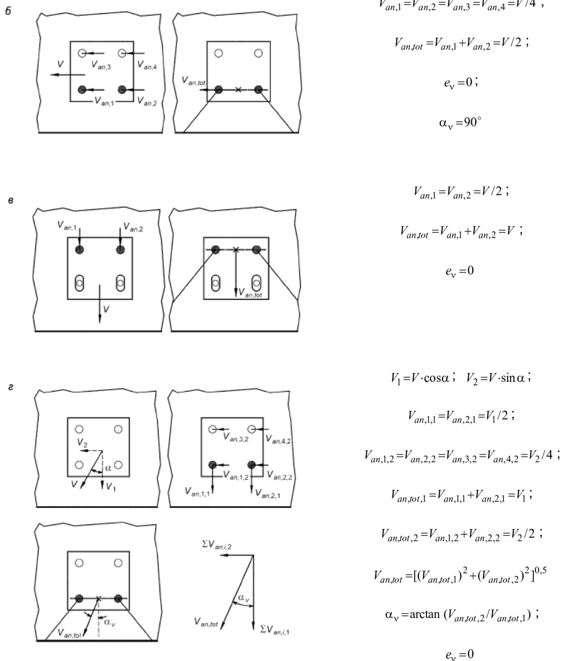
Рисунок 6.8 - Примеры распределения сдвигающих усилий в анкерной группе для расчетов при откалывании края основания
