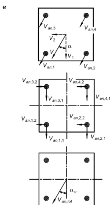
Рисунок 6.7 - Примеры равномерного распределения сдвигающих усилий в анкерной группе
